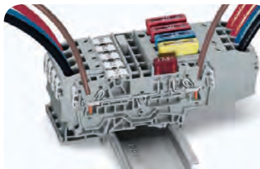
2 yada 4 kablo bağlantılı otomotiv tipi sigortalı klemens
