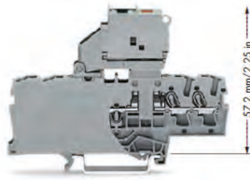
2 yada 4 kablo bağlantılı sigortalı klemens
